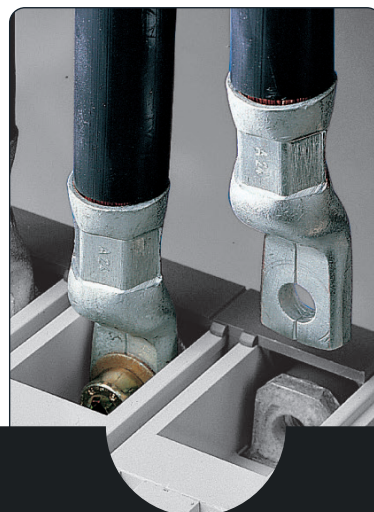
Kabelschuhe
